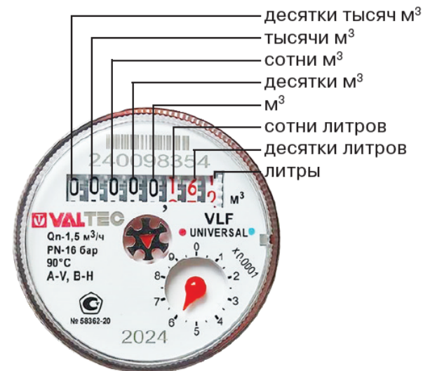
Рис. 3. Табло счетчика
